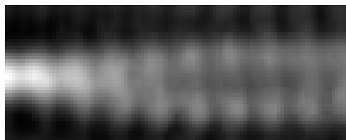
(b) Y Projection
