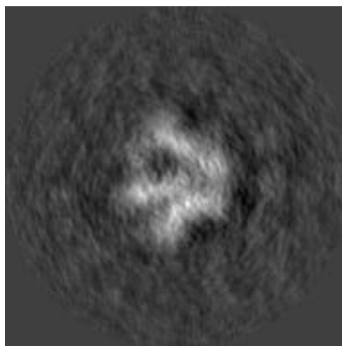
(b) Y Slice 107
