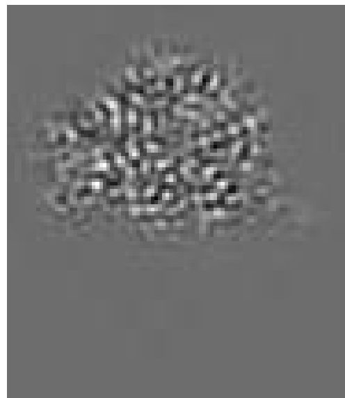
(b) Y Slice 73
