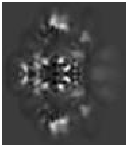
(b) Y Slice 54
