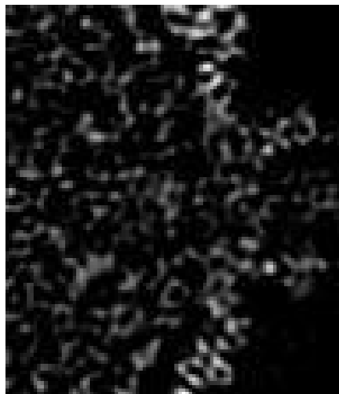
(b) Y Slice 55
