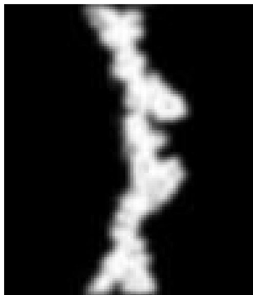
(b) Y Slice 6
