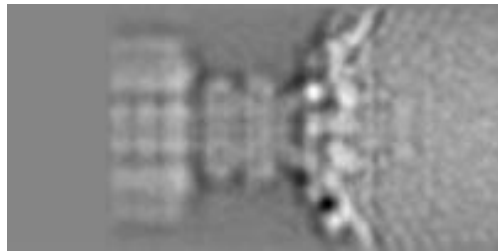
(b) Y Projection
