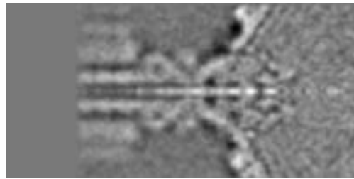
(b) Y Slice 50
