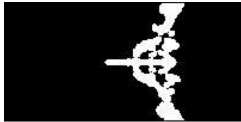
(b) Y Slice 49
